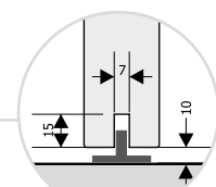
vodící trn
